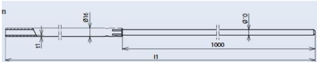
Rysunek techniczny
